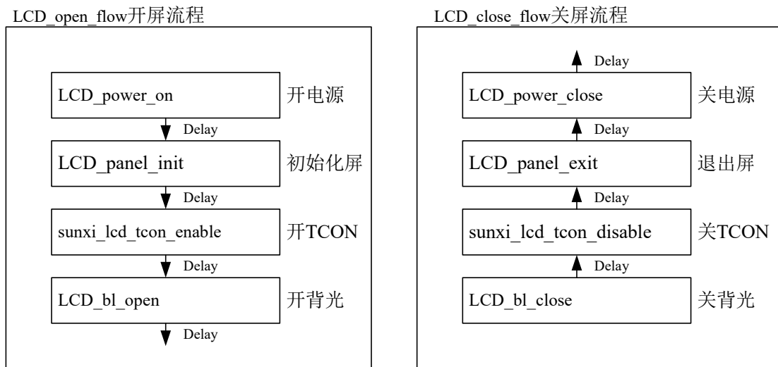
图 6-1 开关屏流程
